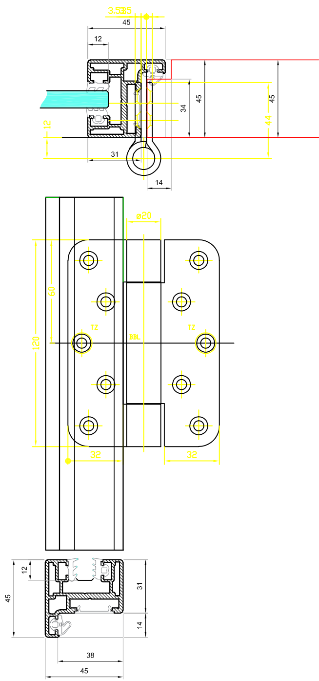
SIMONSWERK VN 2929/120
