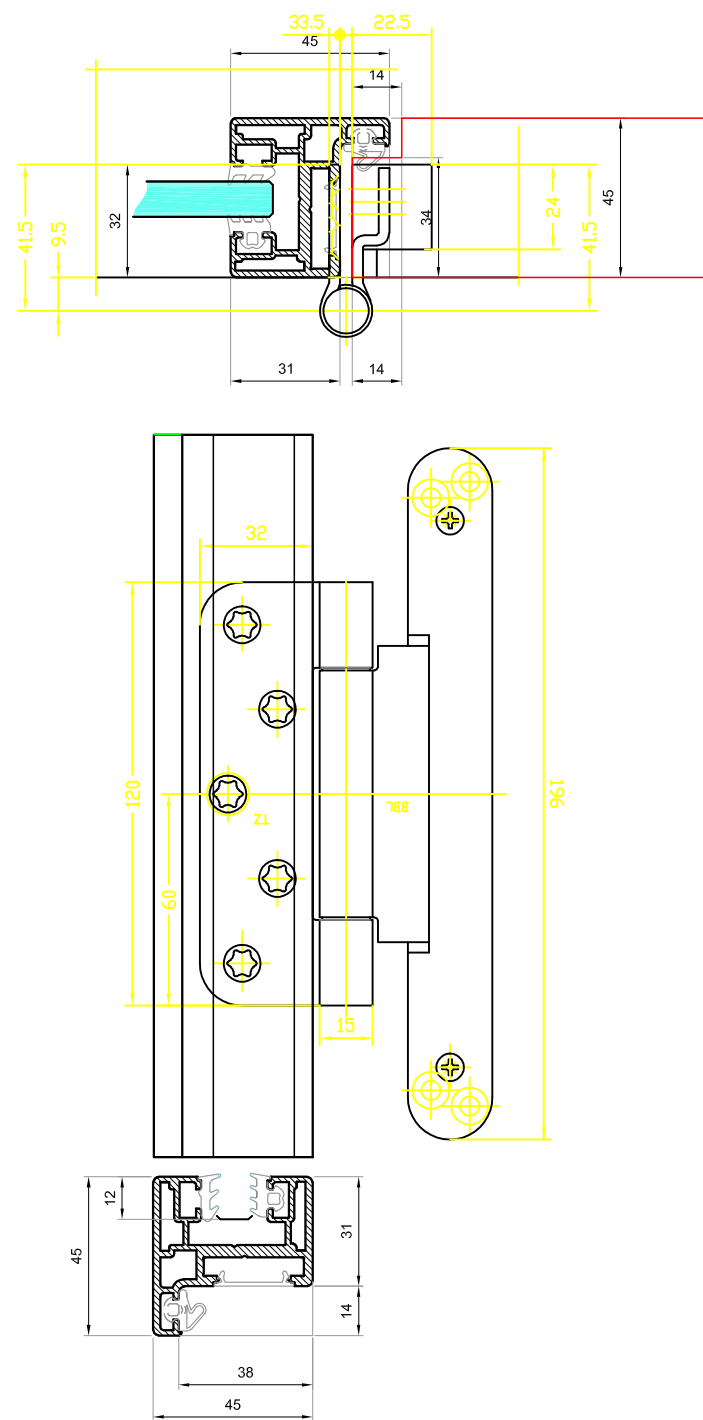
SIMONSWERK VN 2927/120 Compact Planum
